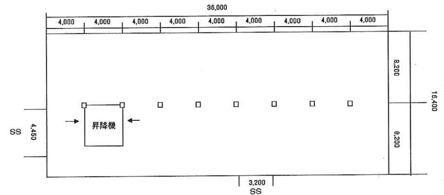
【倉庫1階平面図】
